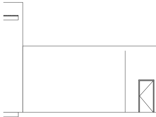
Facade mod øst 1 : 100
